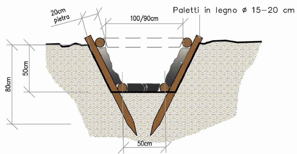
Canaletta di progetto a sezione trapezia
