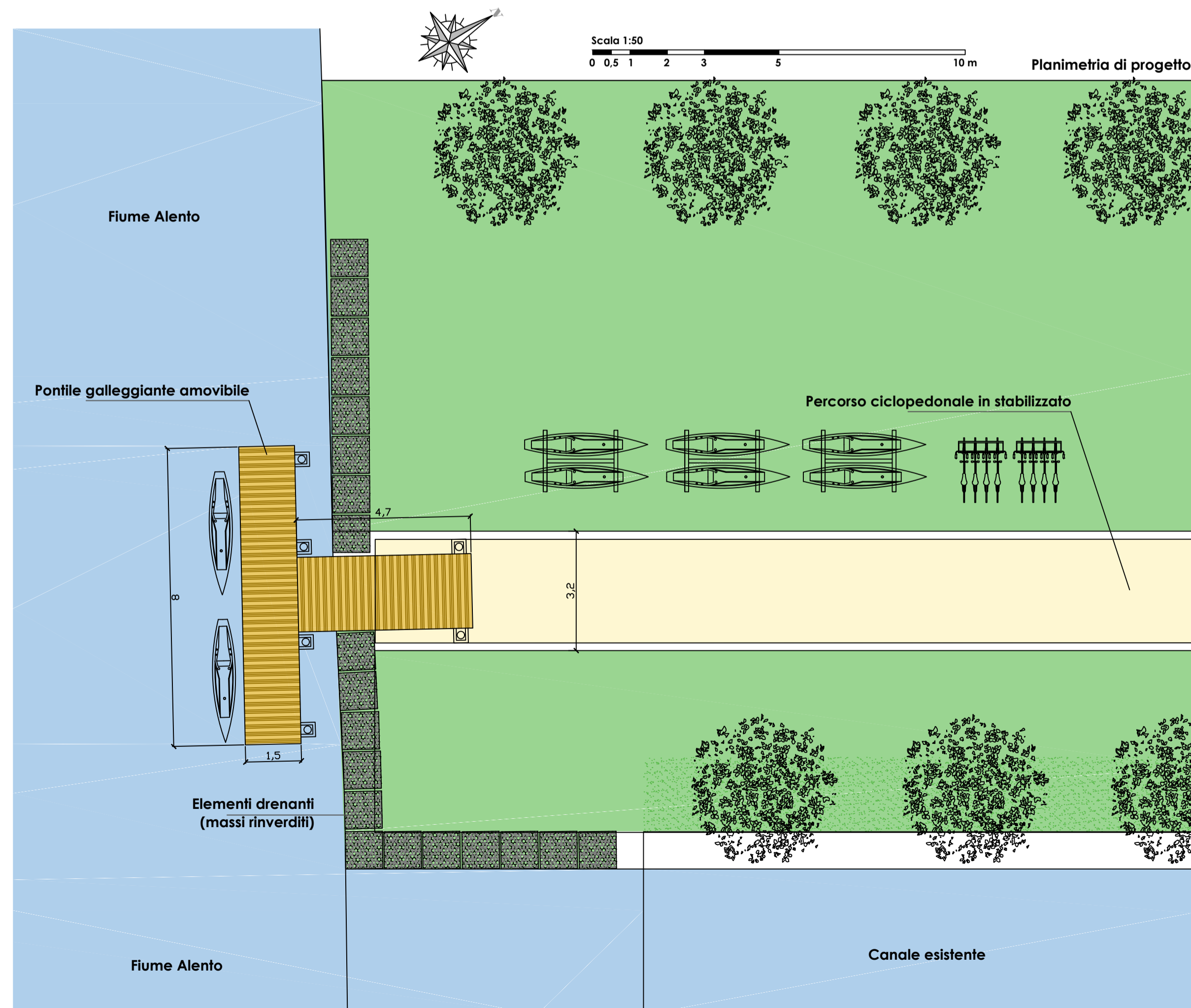
Tipologico molo galleggiante e removibile
