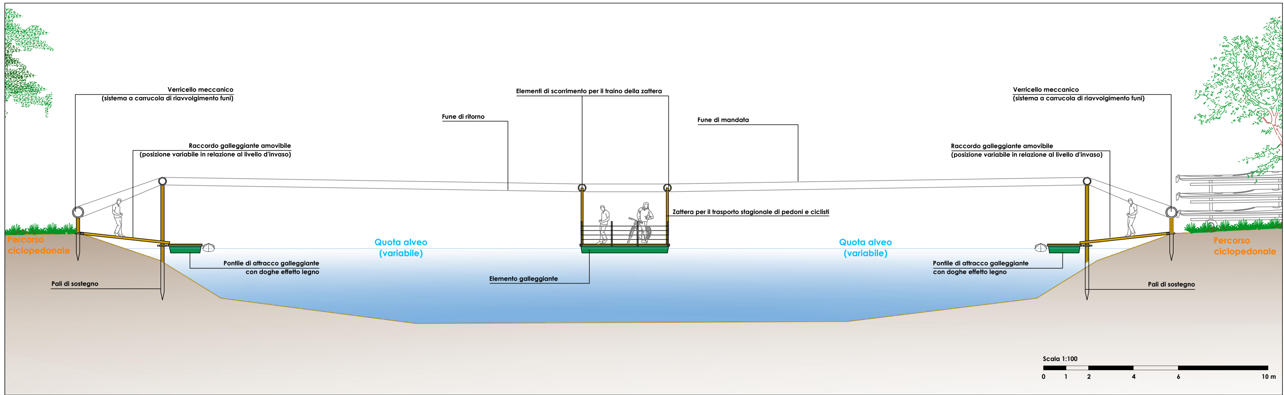
Sistema stagionale e amovibile di attraversamento ciclopedonale dell'alveo fluviale - Sezione tipologica dell'attraversamento (scala 1:100)
