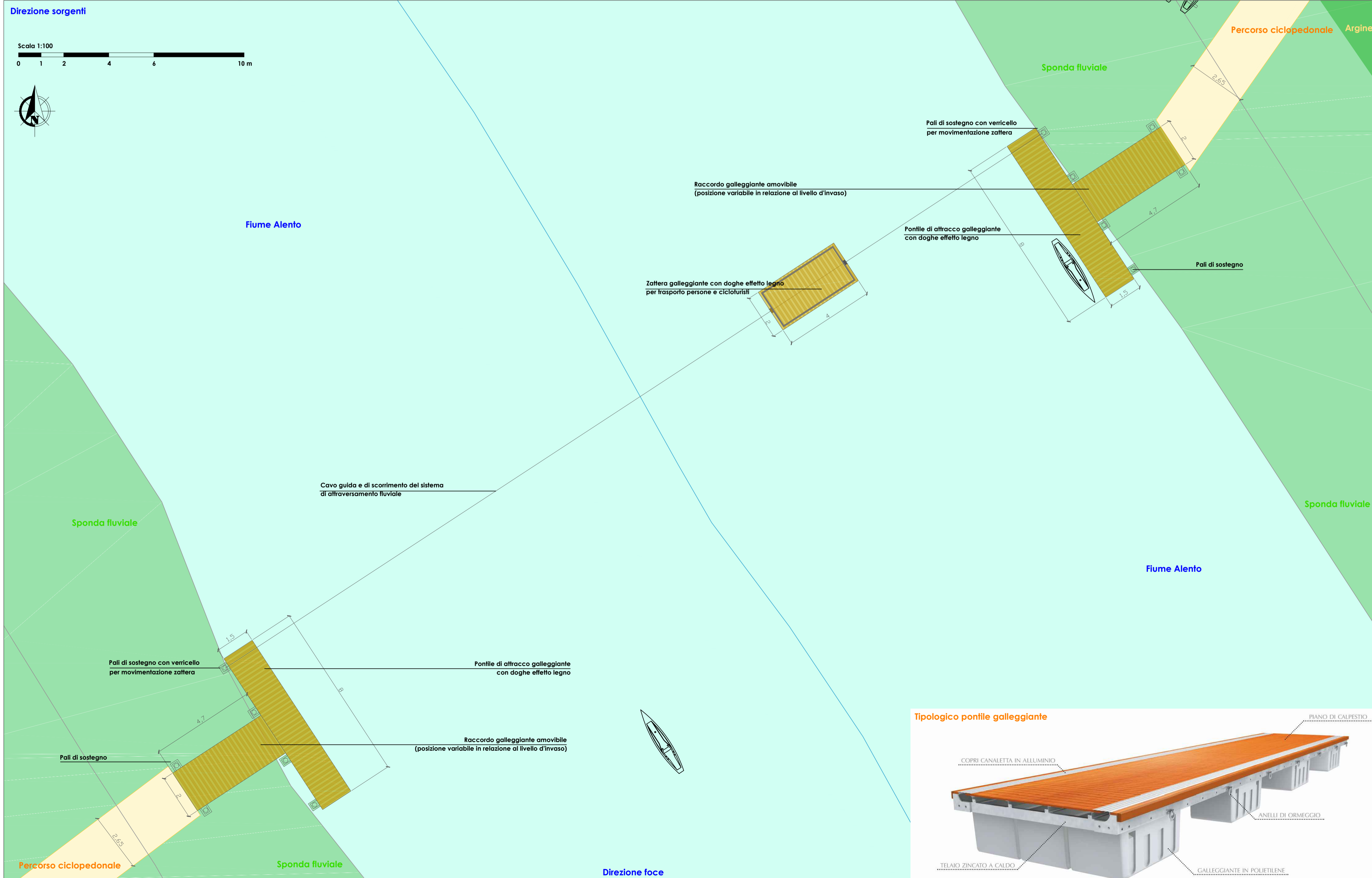
Sistema stagionale e amovibile di attraversamento ciclopedonale dell'alveo fluviale - Planimetria di progetto (scala 1:100)
