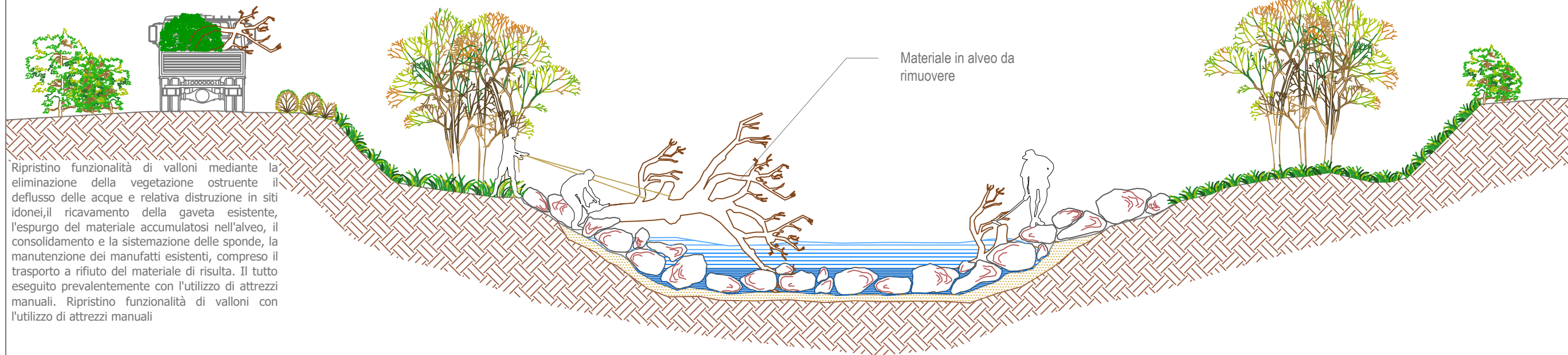
RIMOZIONE MATERIALE IN ALVEO E RIPRISTINO SEZIONE IDRAULICA sezione trasversale corrente... scala 1:100
