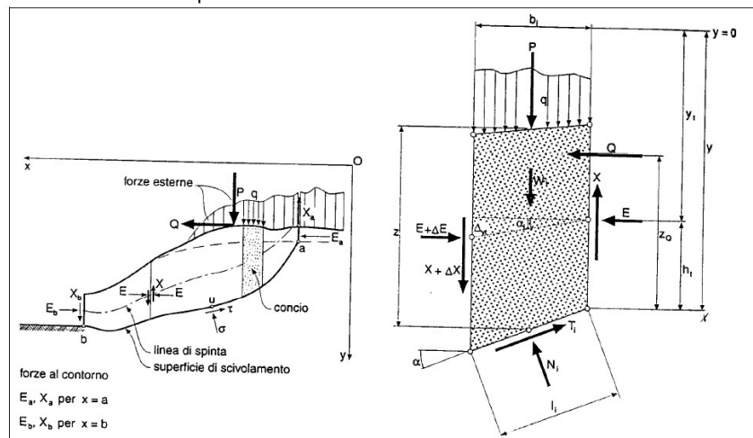
Schematizzazione delle azioni agenti su di un singolo concio
