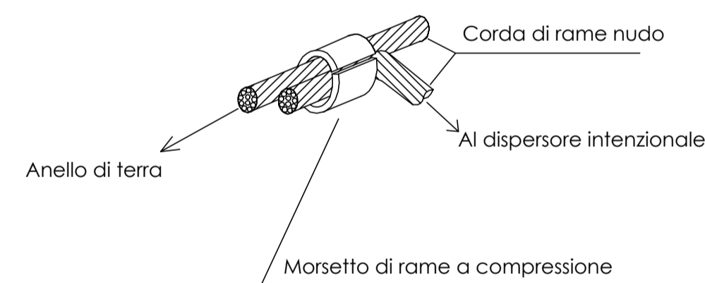
Impianto di terra Giunzione tipica tra corde di rame nudo
